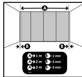
DEHNUNGSFUGENABSTAND
